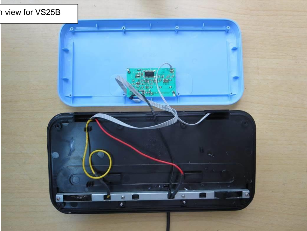
PCB for VS25B and VS25A
